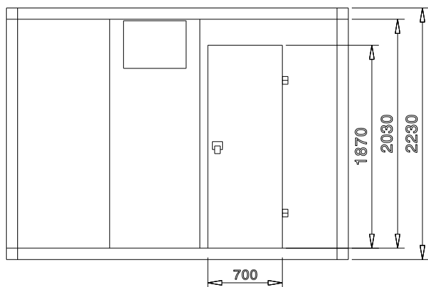
Zij aanzicht
