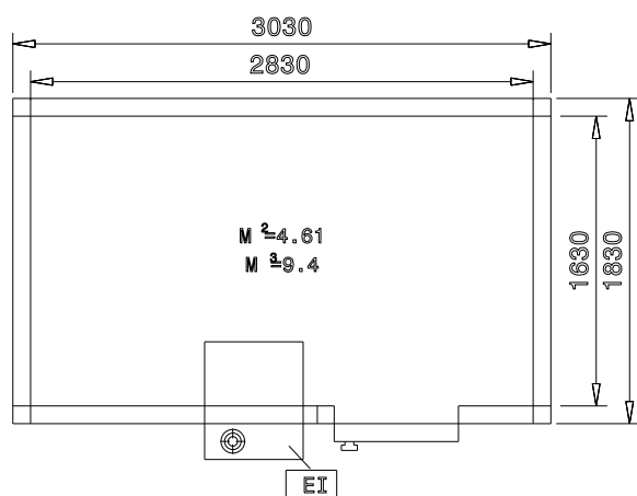
Zij aanzicht
